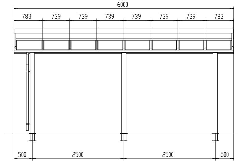
Vorderansicht
